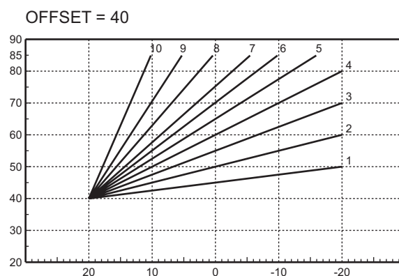
рис. 12 - Пример параллельного смещения компенсационных характеристик
